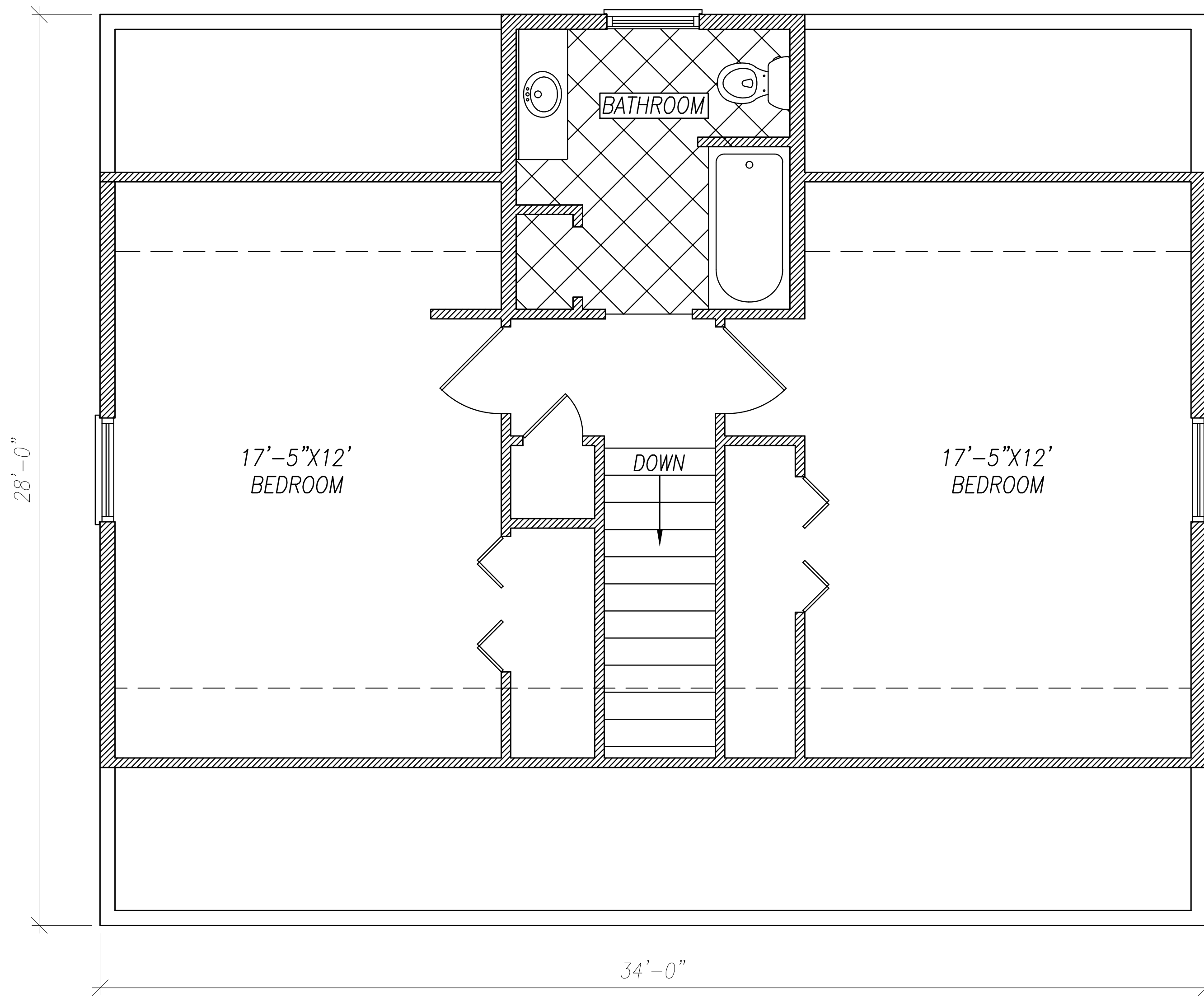
1 FL-2-WALLS Scale: 1:1
